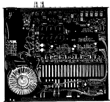
■内部:左下に電源トroidalトランス、右上側が一枚基板上に組み上げられた電源部、増幅部。経路の短縮が図られている。
